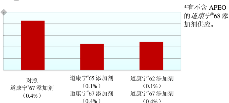
图7：例，凸版印刷油墨配方中采用道康宁® 67 添加剂作为表面活性剂时的消泡性能（添加剂加入量为 0.4%（w/w））。消泡剂的用量仅为 0.1%（w/w，以整个配方为基准）。高速剪切处理后测量泡沫高度，加入道康宁® 62 添加剂或 65*添加剂后，泡沫高度明显减小。
