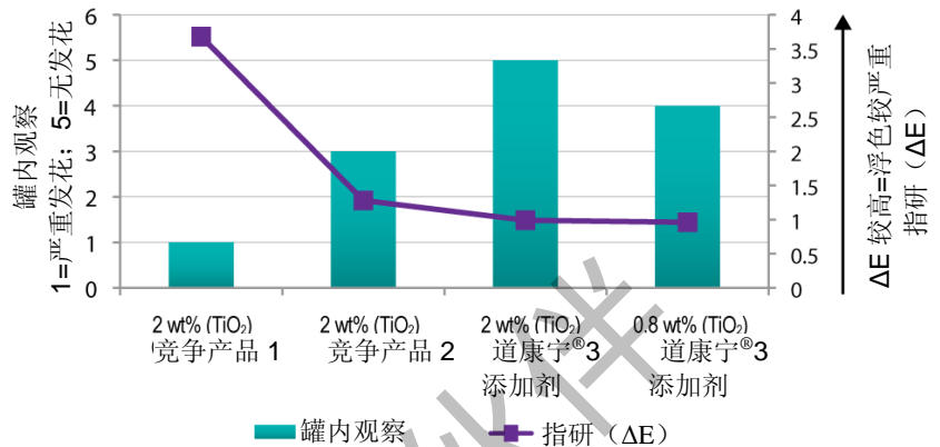
图3: 一种溶剂型 2K 聚氨酯 (PU) 灰色木器涂料中的发花 (罐内观察) 和浮色现象 (指研结果)。如图所示, 通过后添加所示添加量的道康宁® 3 添加剂和竞争产品 2, 性能明显提升。
