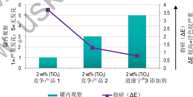
图 1: 道康宁® 3 添加剂与竞争分散剂产品在一种溶剂型 2K 聚氨酯 (PU) 灰色木器涂料中的发花（罐内观察）和浮色现象（指研结果）对比。所有添加剂均在白色基料研磨时添加。
